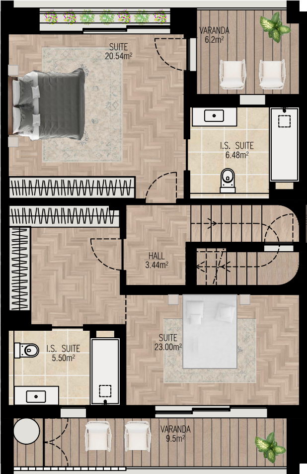
Planta piso 1
