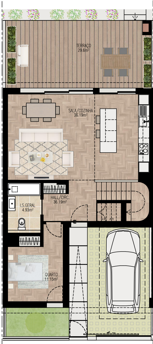
Planta piso 0
