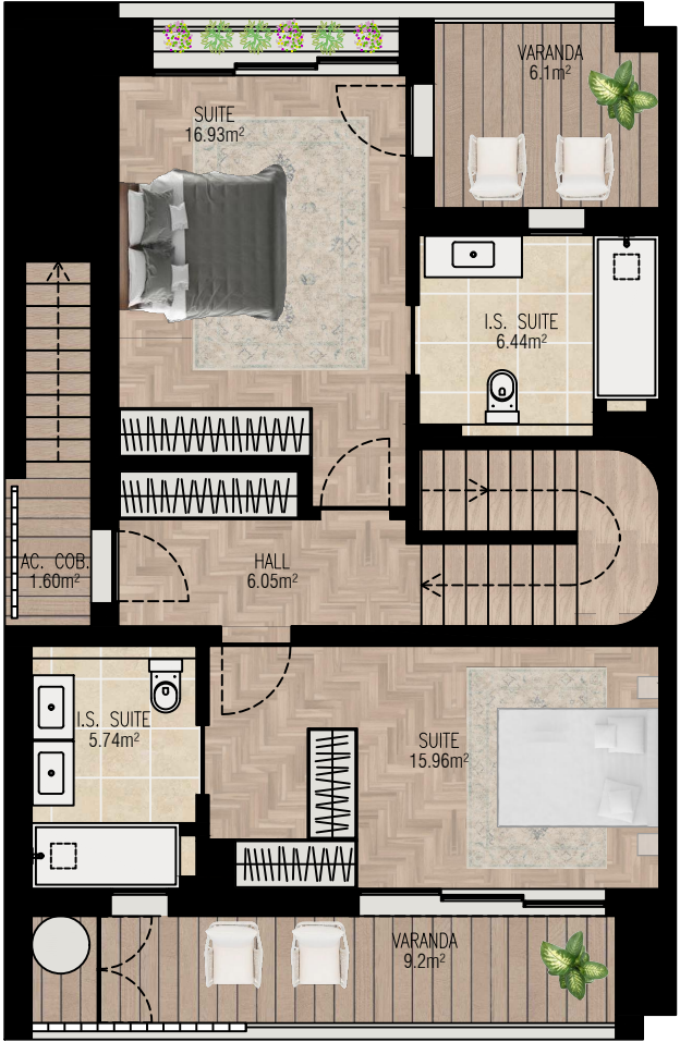
Planta piso 1
